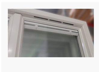
Utsidan Epok Fräsning för ventilen i Epokkarmen visas på bilden. På samma sätt för Royalkarmen. Dvs dolt luftintag för Epok- och Royalmodellen.
