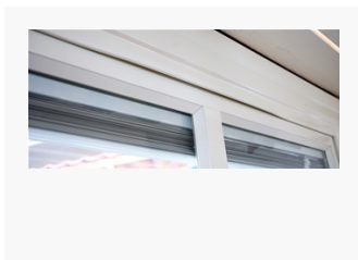
Utsida Haga Utsida av ventil för öppningsbart fönster av modell Haga. Aluminiumkarmen har en utbökning för ventilens luftintag.
