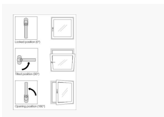
Hoppe TBT TBT-tekniken möjliggör låsning av handtaget med en nyckel med lutning (90°-position). Handtaget kan vridas vidare till öppningspositionen (180°-position) enbart efter upplåsning med nyckeln.
